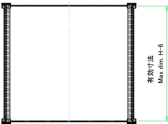
Wパネル1 / W Panel 1
